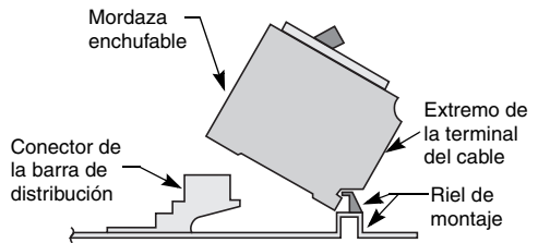
Figura 5: Interruptor automático derivado Homeline
