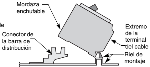
Figura 7: Interruptor automático en tándem Homeline
